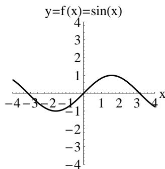
Sine Function
